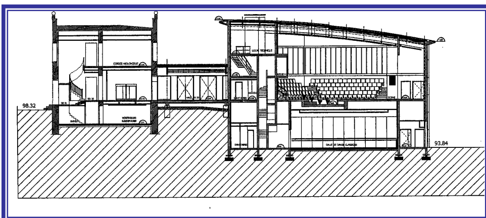
Coupe longitudinale
