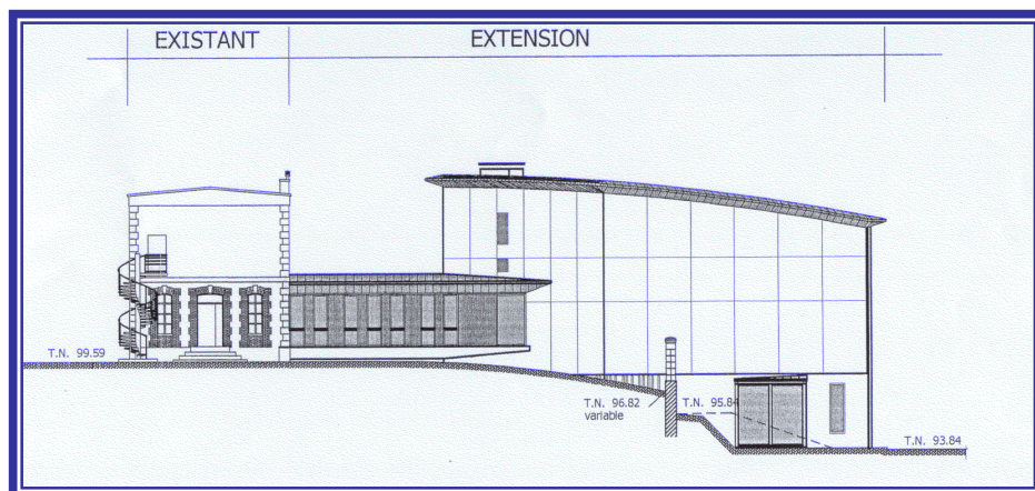
Coupe sur terrain naturel
